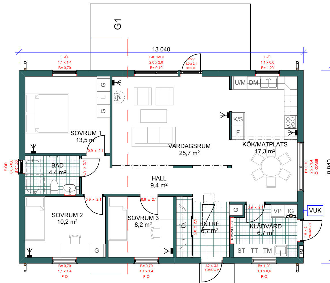
LYCKAN 2 ENTRÉVÅNING 103,4 m 2 BOA, 115,3 m 2 BYA
