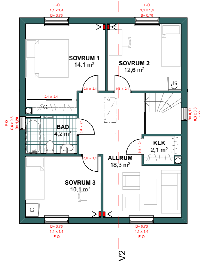
ÖVERVÅNING 65,1 m 2 BOA
