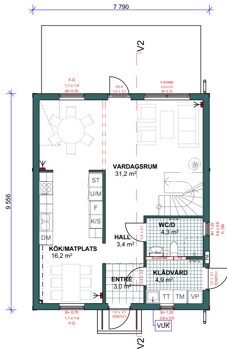
GLÄDJEN 1 ENTRÉVÅNING 65,1 m 2 BOA, 74,4 m 2 BYA
